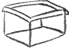
Tupperware
